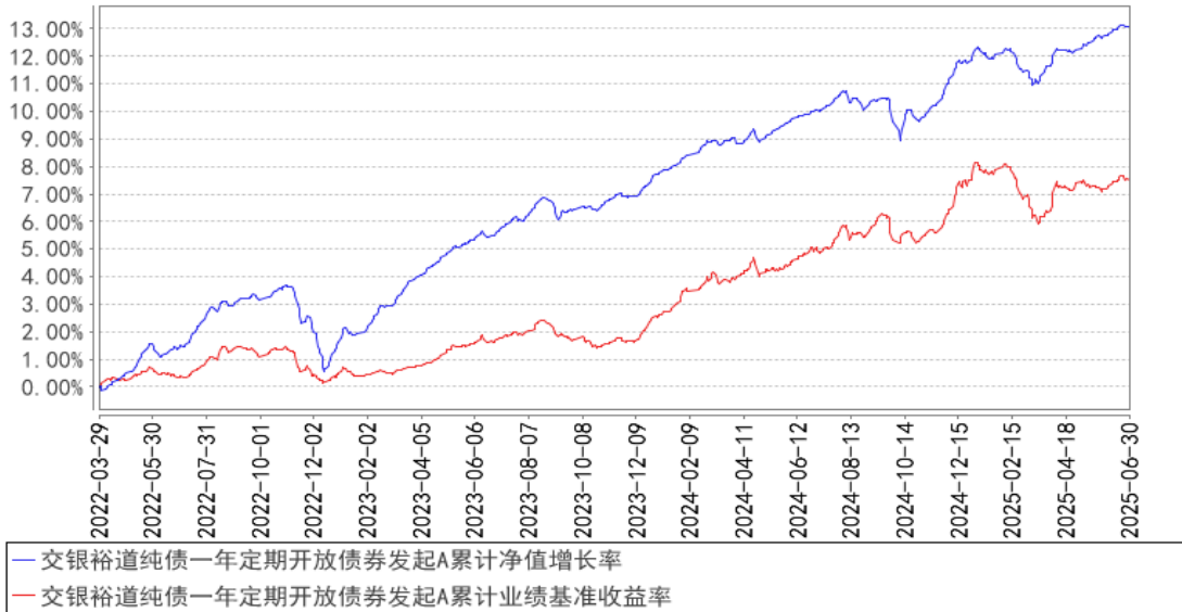
交银裕道纯债一年定期开放债券发起A累计净值增长率与同期业绩比较基准收益率的历史走势对比图
