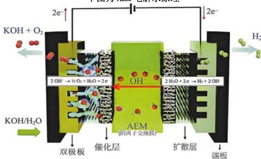
下图为 AEM 电解水原理
