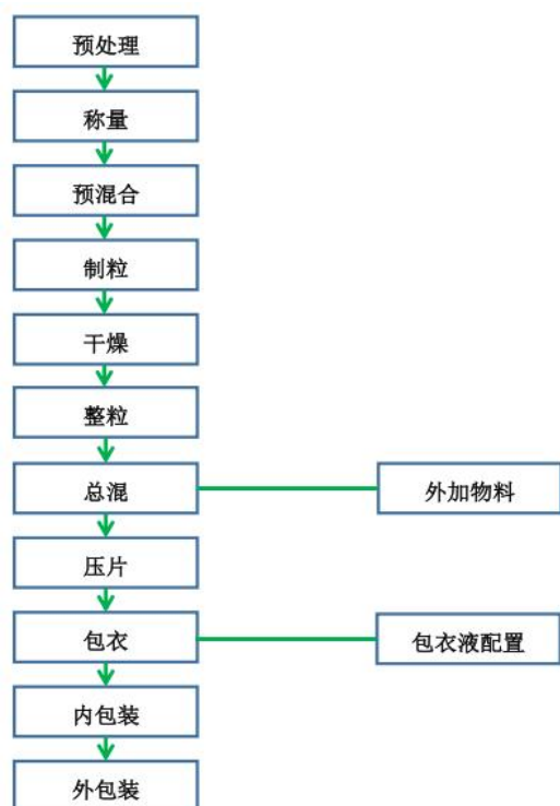
片剂生产工艺流程图
