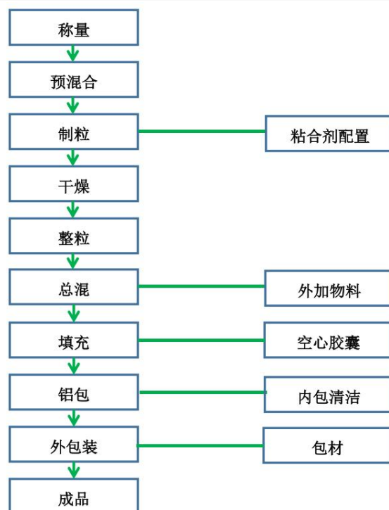
胶囊剂生产工艺流程图
