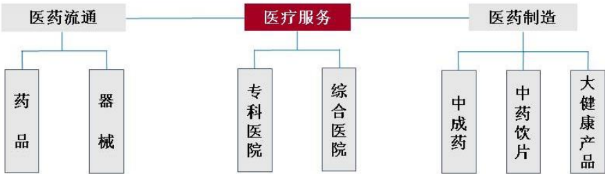
业务架构
