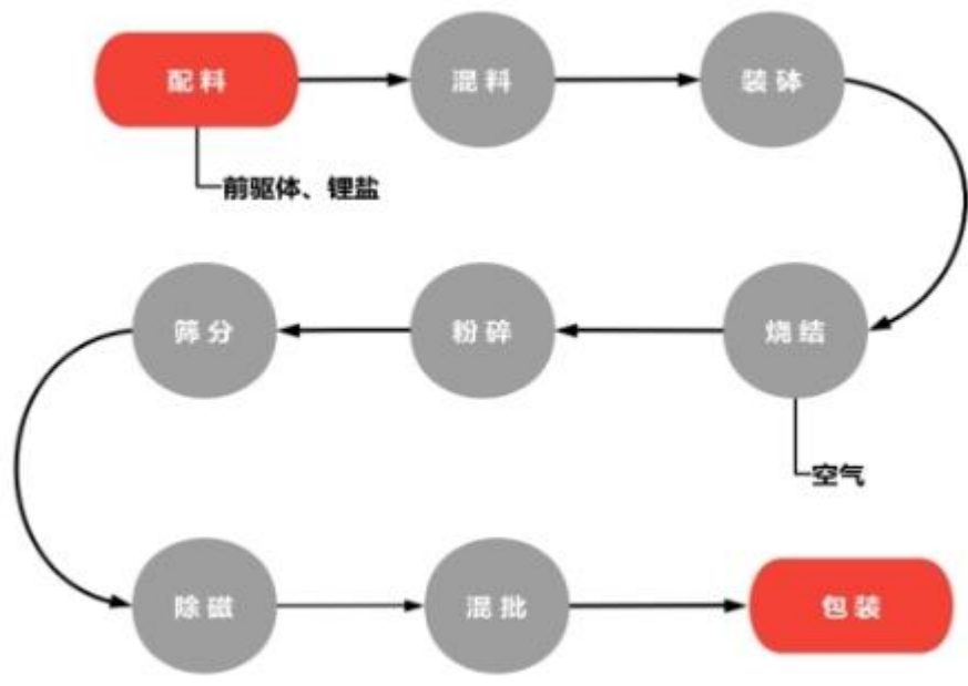
(3) 高镍三元材料工艺流程:
