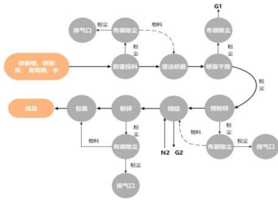
(2) 常规三元材料工艺流程:
