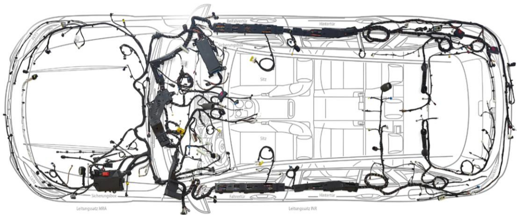
汽车线束车内布局结构示例 1，图例来源：LEONI
