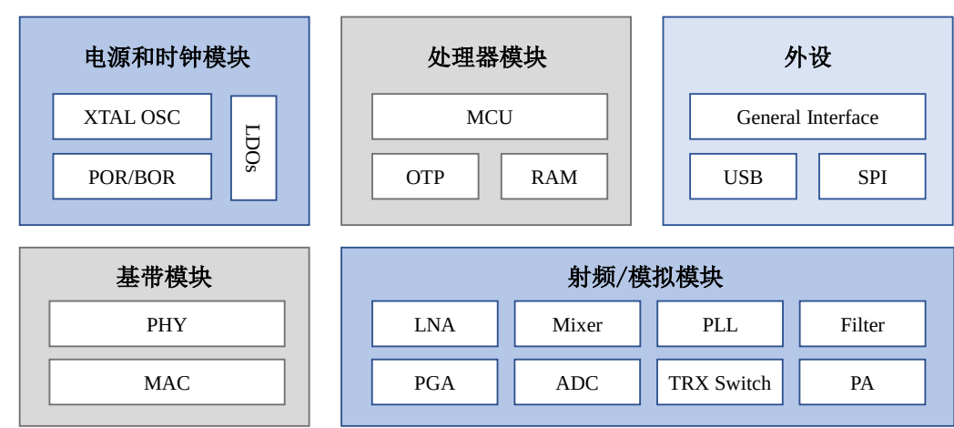
2.4G 私有协议类 SoC 芯片架构
