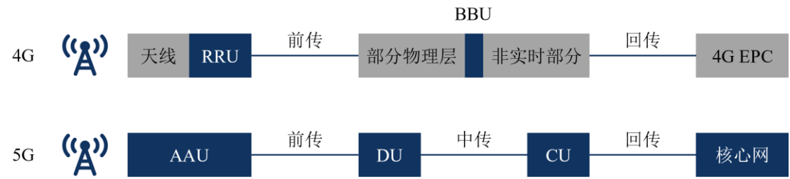
移动通信基站结构
