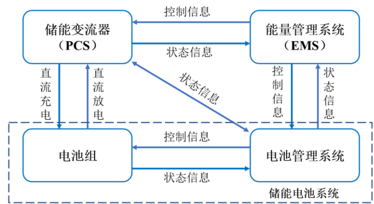
电化学储能系统主要构成
