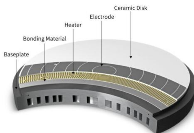
图：静电吸盘结构示意图
