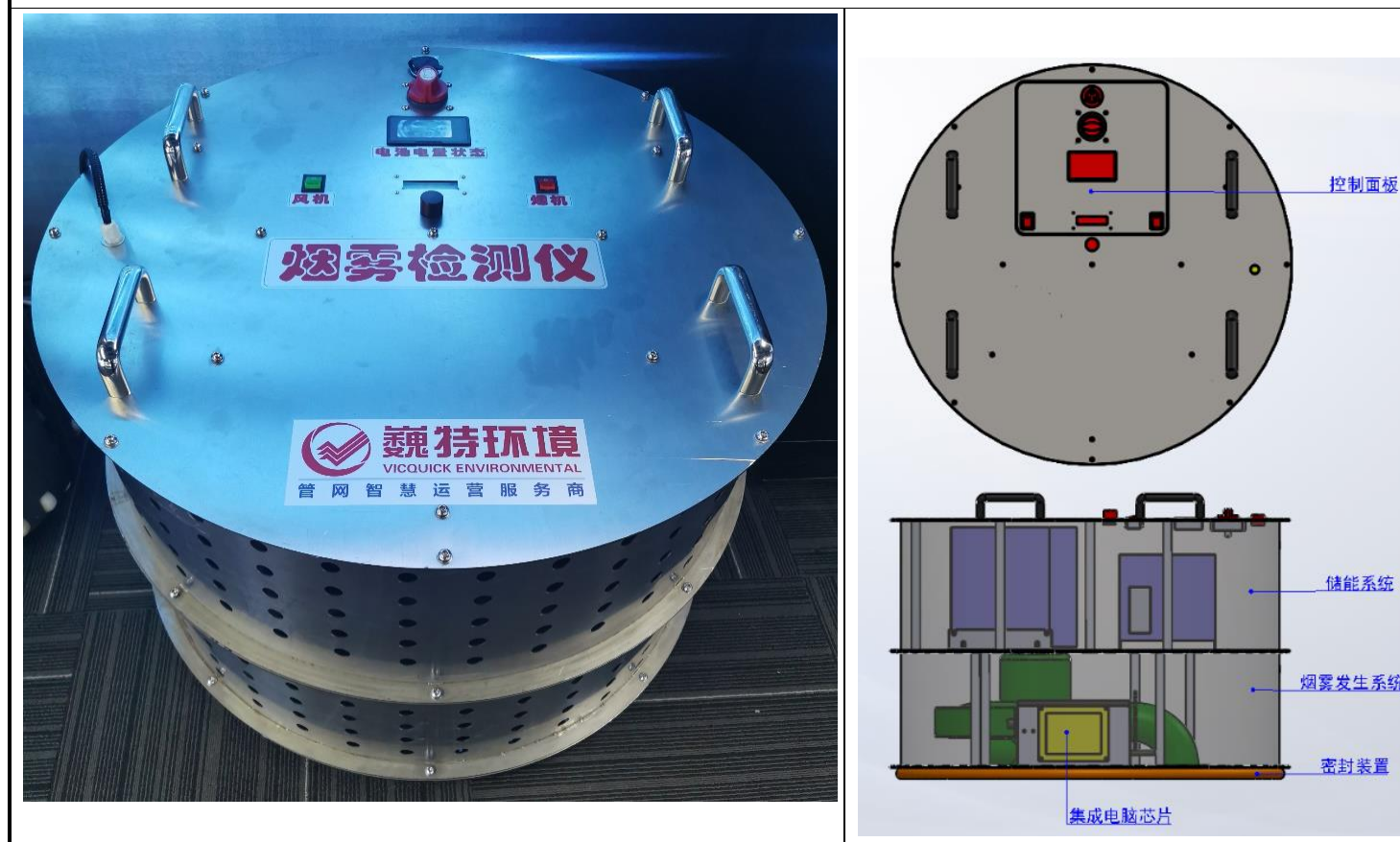
发行人研发的烟雾检测仪器示意图
