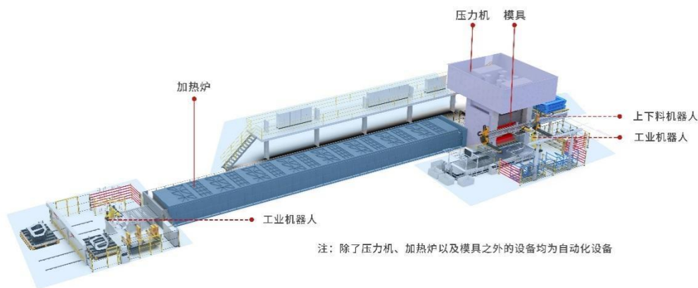
上图为一完整的热冲压自动化生产线
