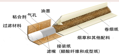
传统卷烟拆解图
