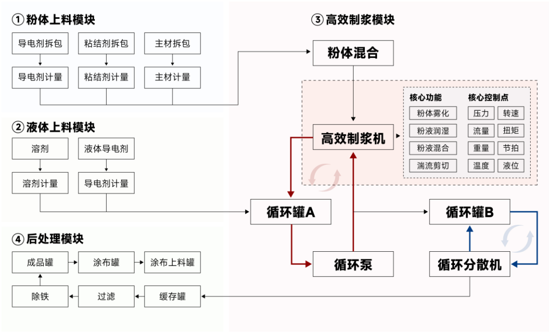
循环式高效制浆系统工艺流程图
