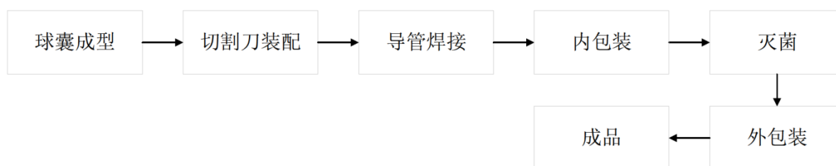
切割球囊扩张导管生产工艺流程图
