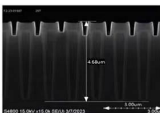
更新一代自对准结构
