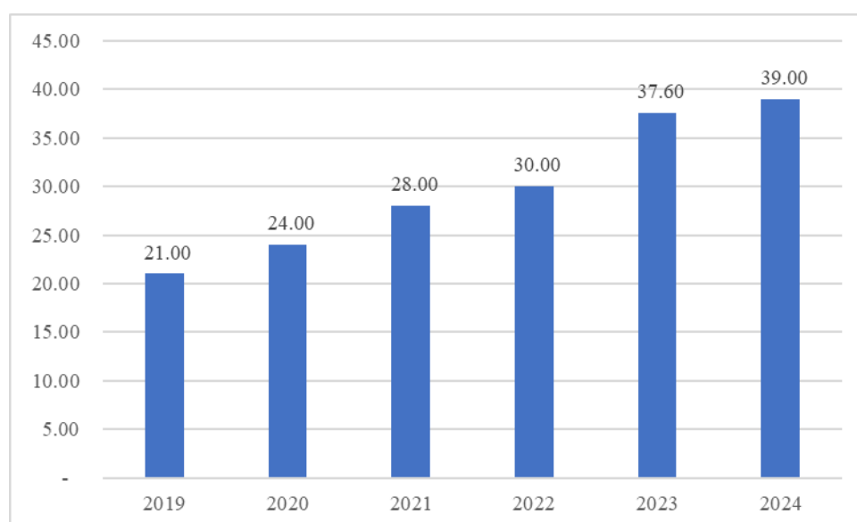
2019-2024 年全球稀土产量（万吨）
