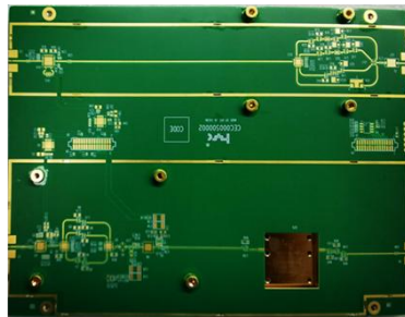
4层铜基基板
