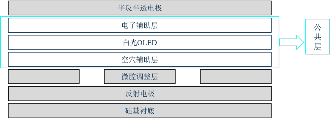
硅基 OLED 强微腔结构示意图
