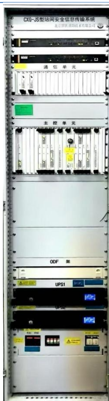
CXG-JS 型站间安全信息传输系统机柜
