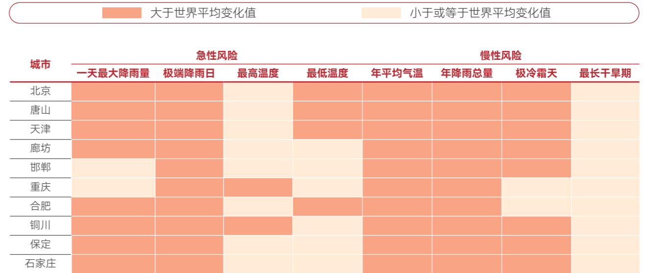
IPCC SSP5-8.5 情景下 2050 年物理风险热力图
