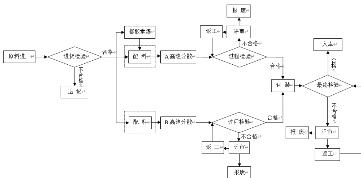
图1 改性丙烯酸酯胶粘剂生产工艺流程图
