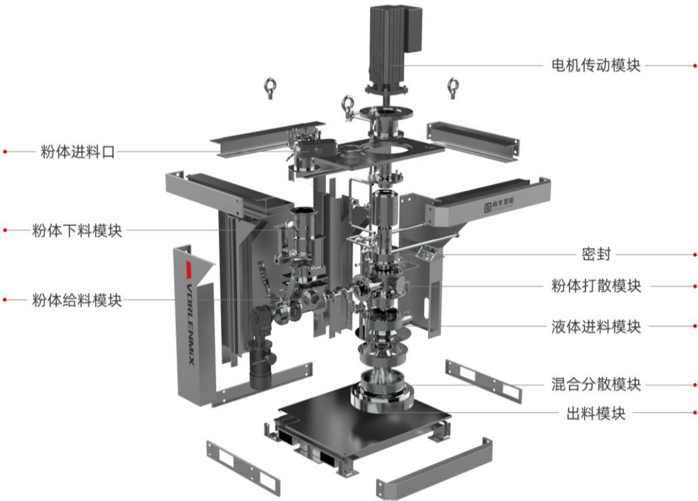
循环式高效制浆机整体架构图
