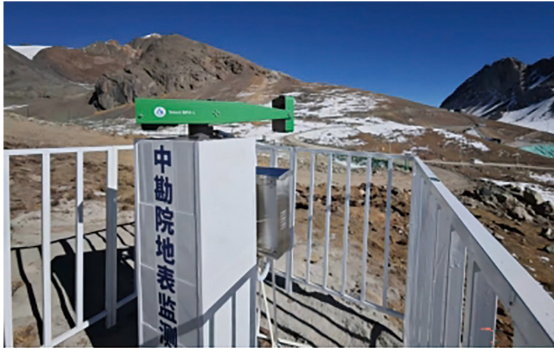
礦山數智安全監測系統
