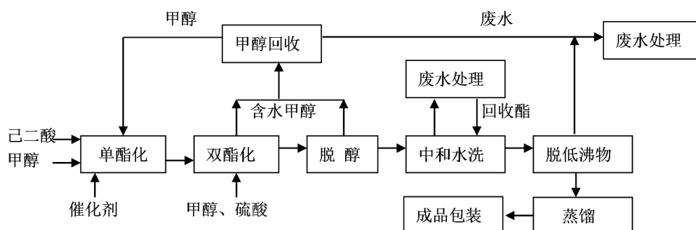
DMA 生产工艺流程图
