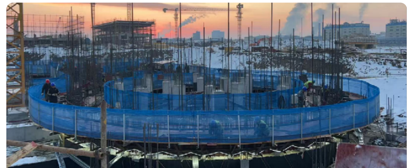
建设中的安徽蚌埠 100 万吨 / 年新型作物专用肥项目
