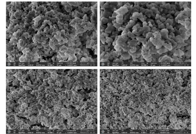
现有批量产品——P 系列磷酸铁（扫描电镜）
