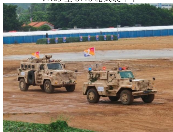
VP11 型 4×4 轻型防地雷装甲车
