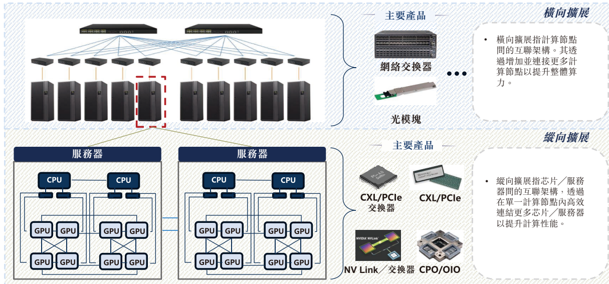
高速互連網路原理圖
