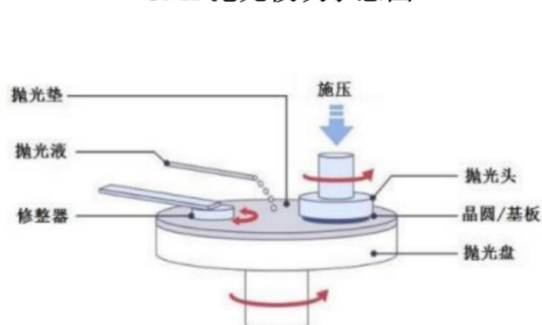
CMP抛光模块示意图
