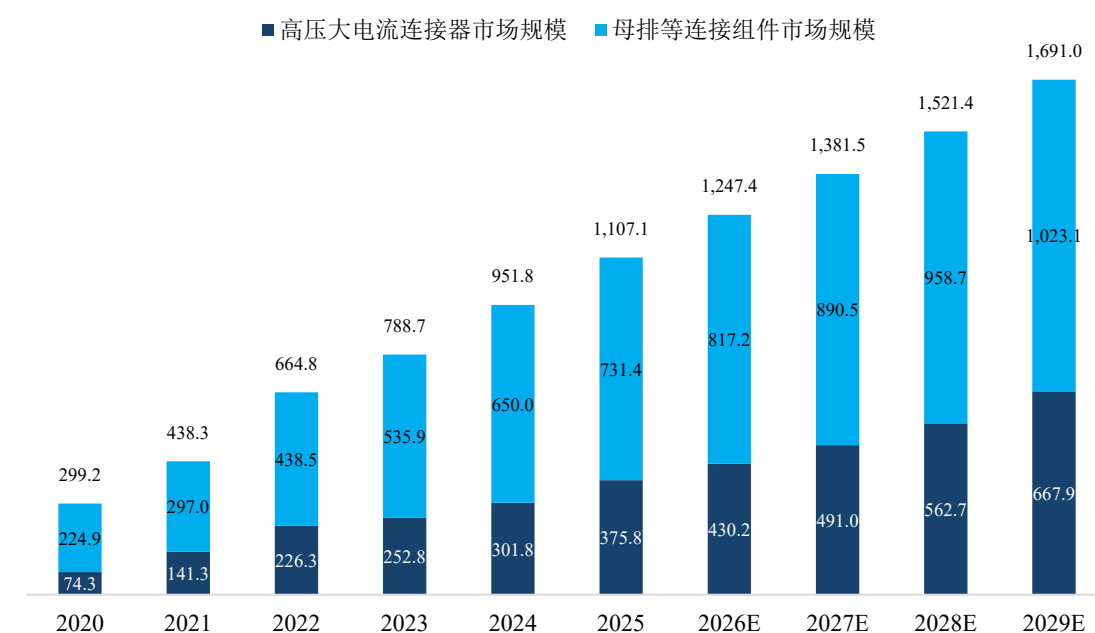
中国高压大电流连接系统市场规模（亿元），2020-2029E
