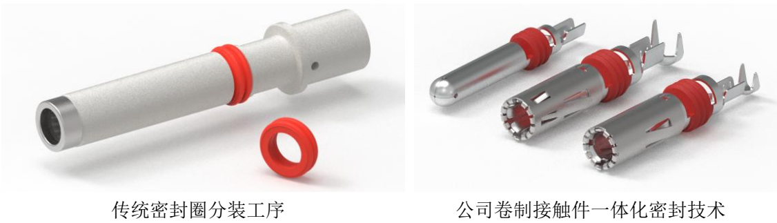
传统密封工序与公司一体化密封技术差异示意图
