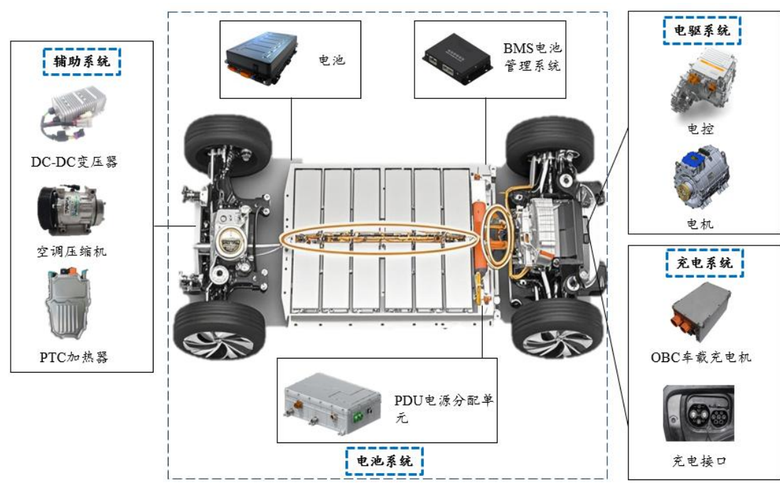
高压大电流连接器在新能源汽车中应用示意图
