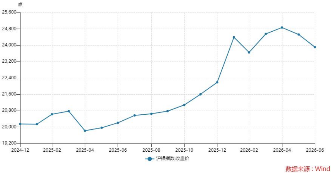
2025 年度至 2026 年上半年铝价走势图（沪铝现货，单位：元/吨）
