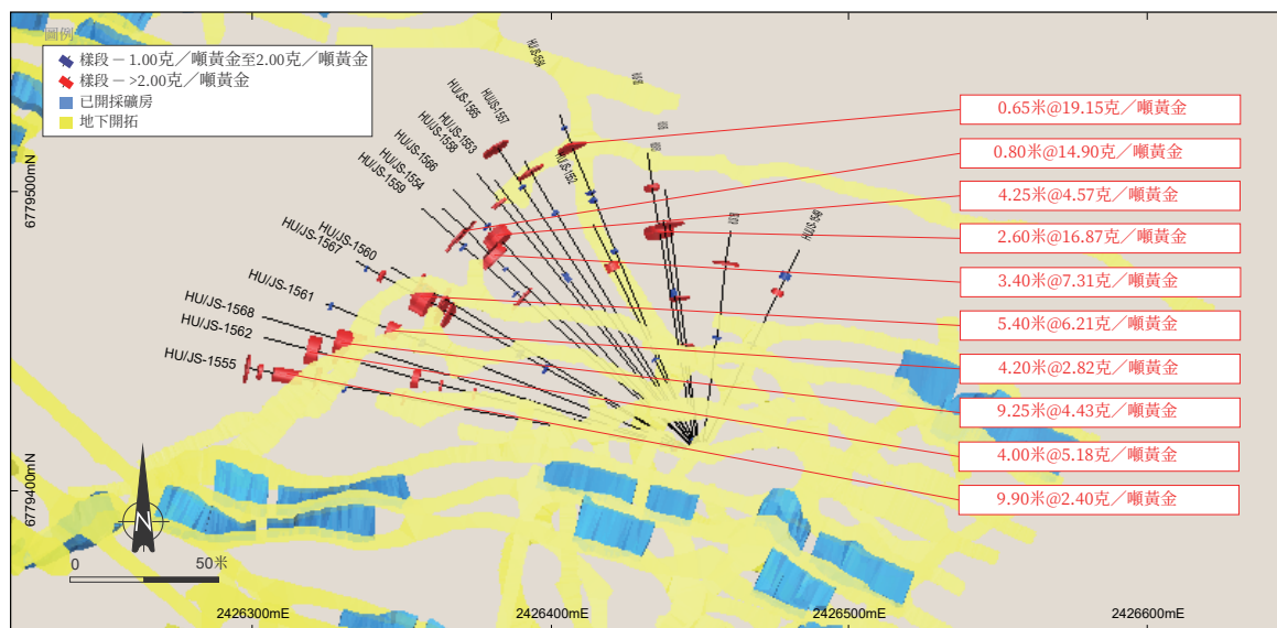
圖4—2026 Arpola-4活動平面視圖，突出顯示 \geq 10 克*米的樣段。
