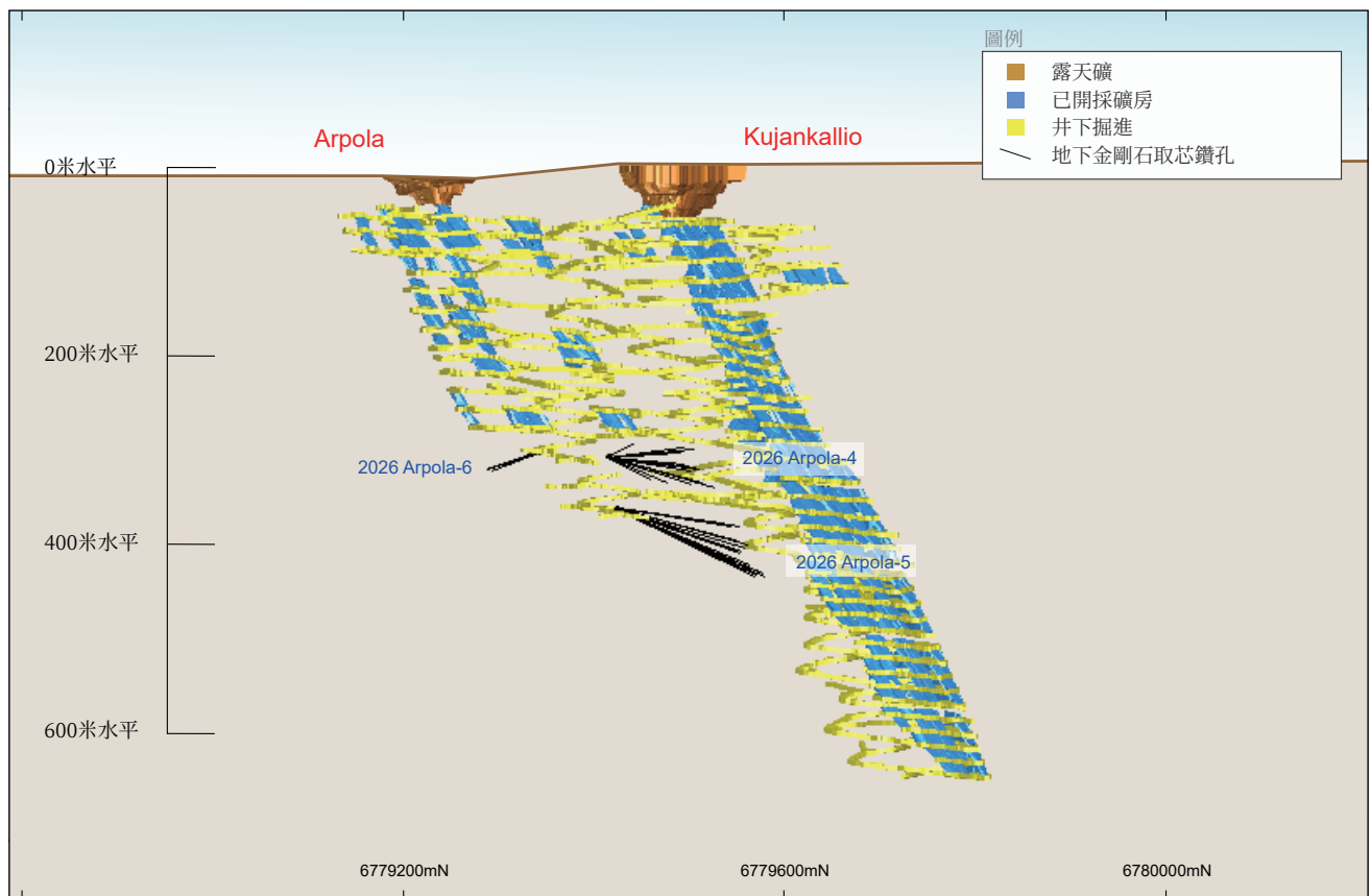
圖3－Jokisivu 金礦顯示報告的鑽探工程位置。向西視圖。
