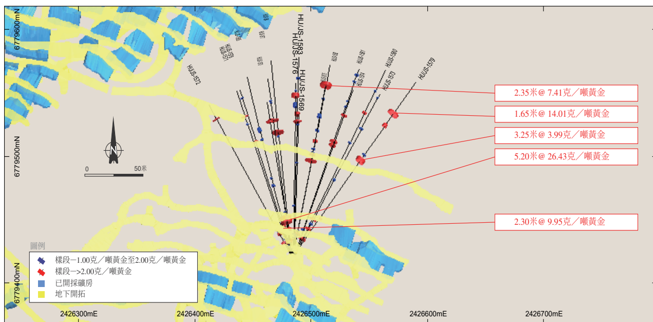
圖5—2026 Arpola-5活動平面視圖，突出顯示 \geq 10 克*米的樣段。
