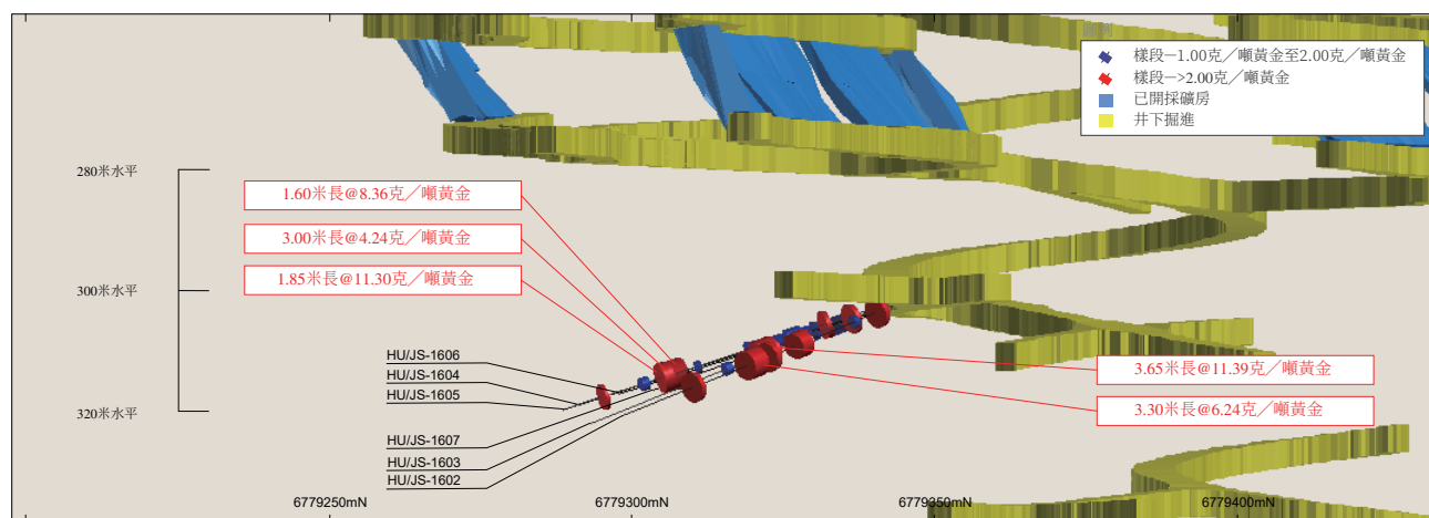
圖6—2026 Arpola-6活動向東俯視圖，突出顯示 \geq 10 克*米的樣段。
