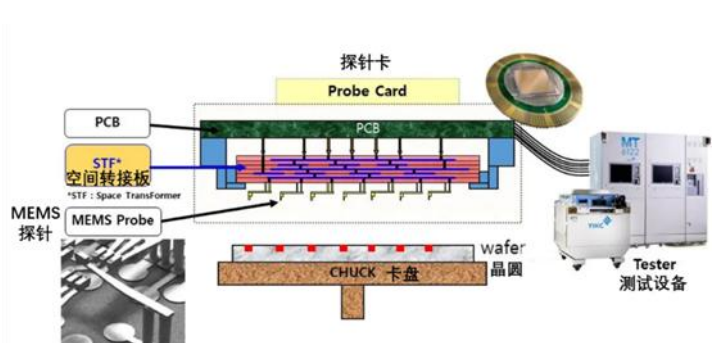
图：探针卡 来源：国金证券
