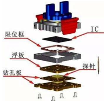
图：IC 测试座结构示意图 来源：国金证券
