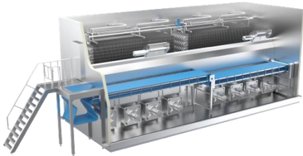
流态化速冻装置
