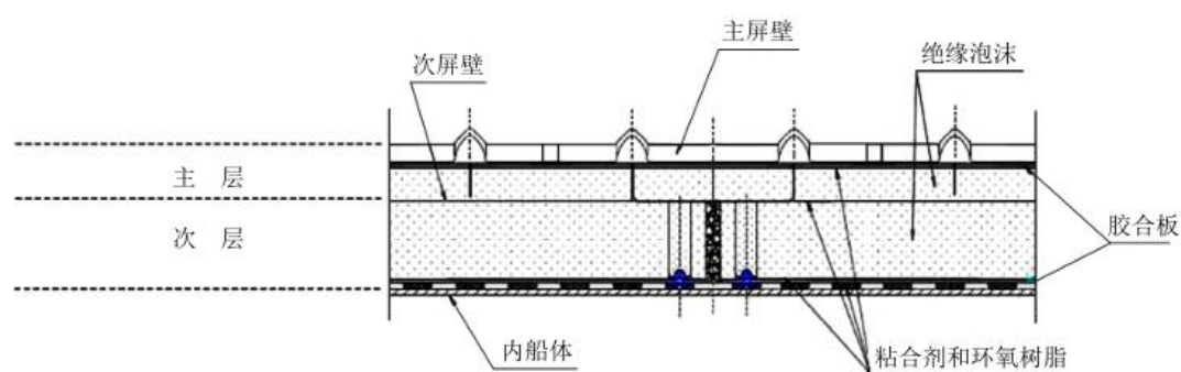
图 MARKIII FLEX 型围护系统典型剖面
