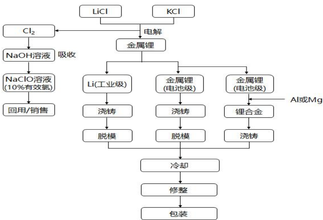
(3) 金属锂生产工艺流程图
