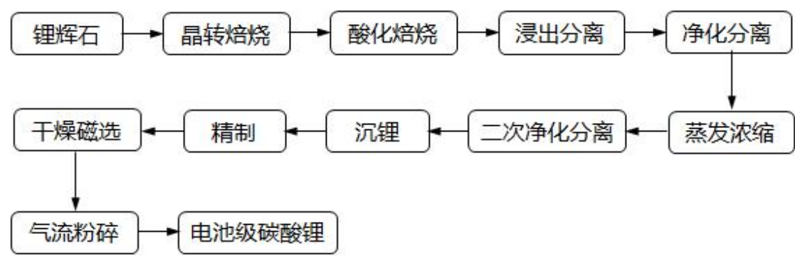
(2) 氢氧化锂生产工艺流程图
