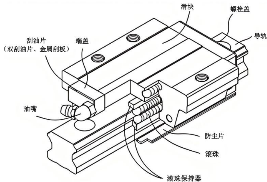
直线导轨副结构示意图
