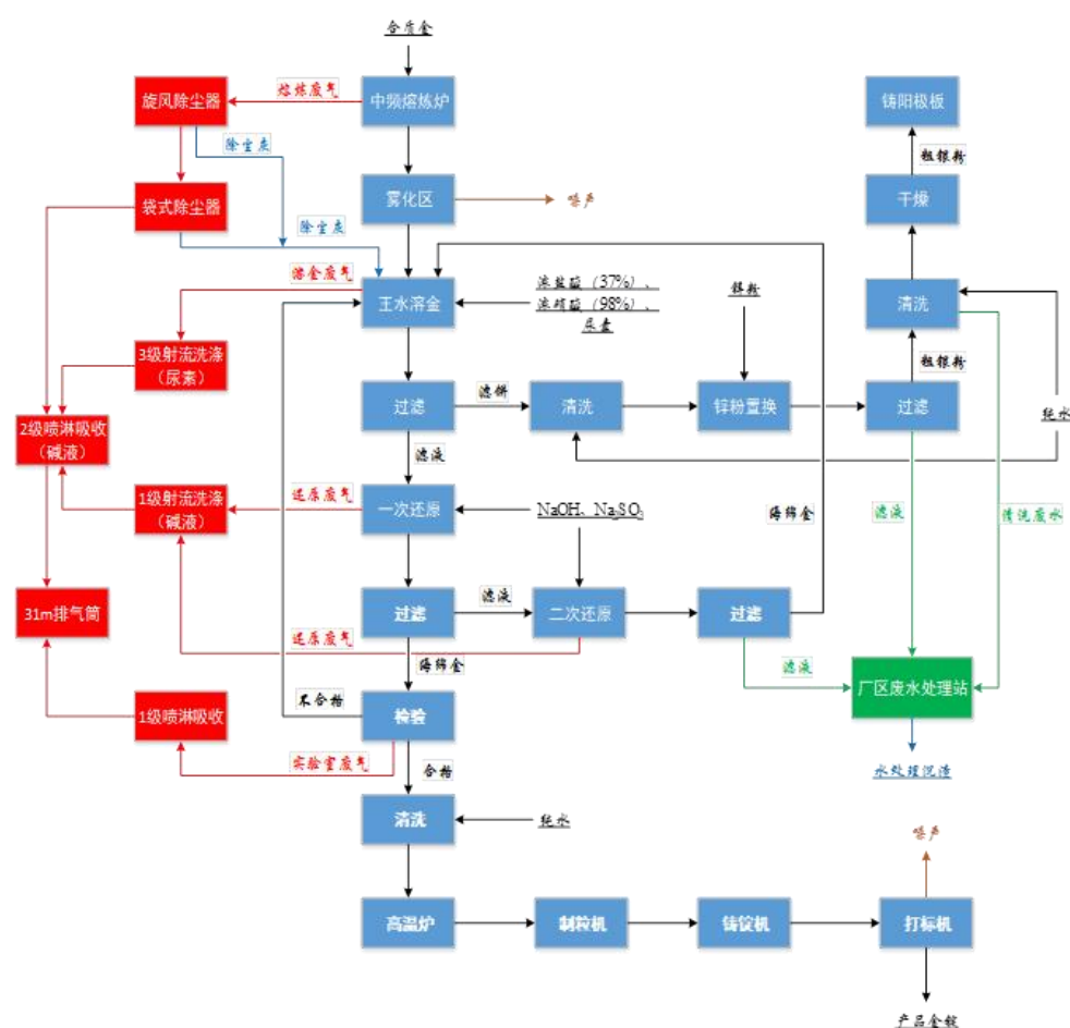
图表 5-15：工艺流程图
