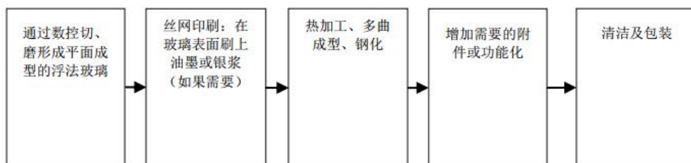
图表5-8-9 汽车玻璃生产工艺流程图
