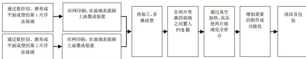
图表5-8-8 夹层汽车玻璃生产工艺流程图
