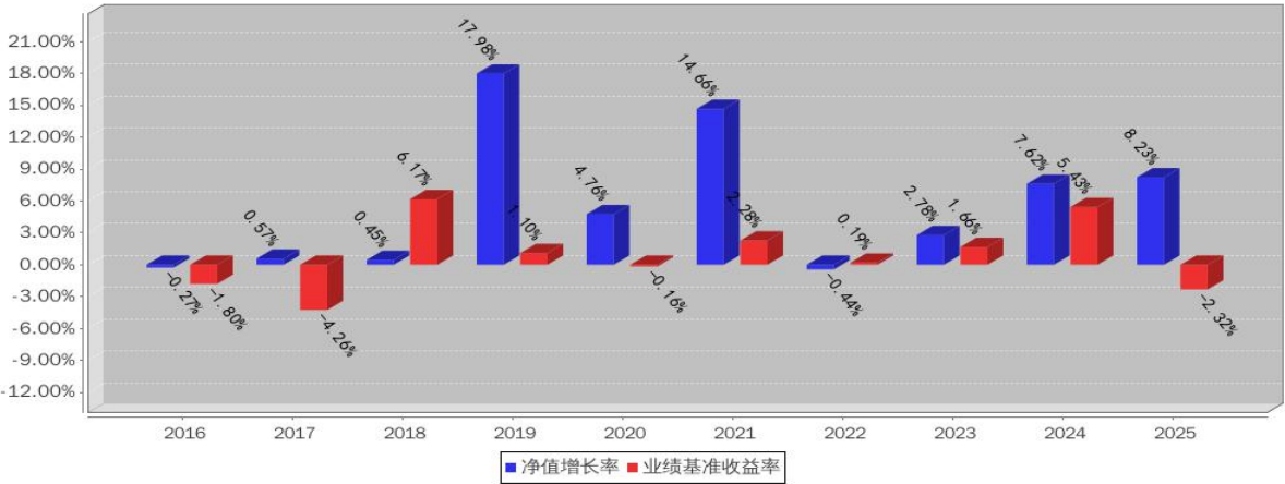
万家添利C基金每年净值增长率与同期业绩比较基准收益率的对比图（2025年12月31日）
