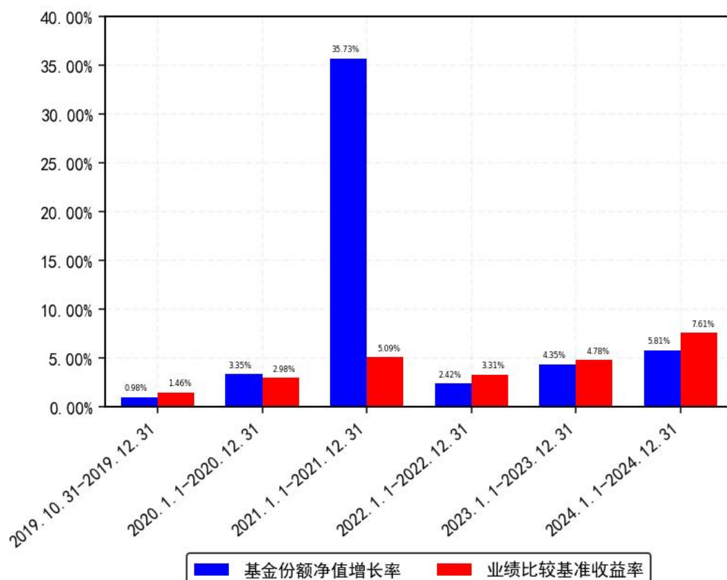
招商招华纯债C每年净值增长率与同期业绩比较基准收益率的对比图
