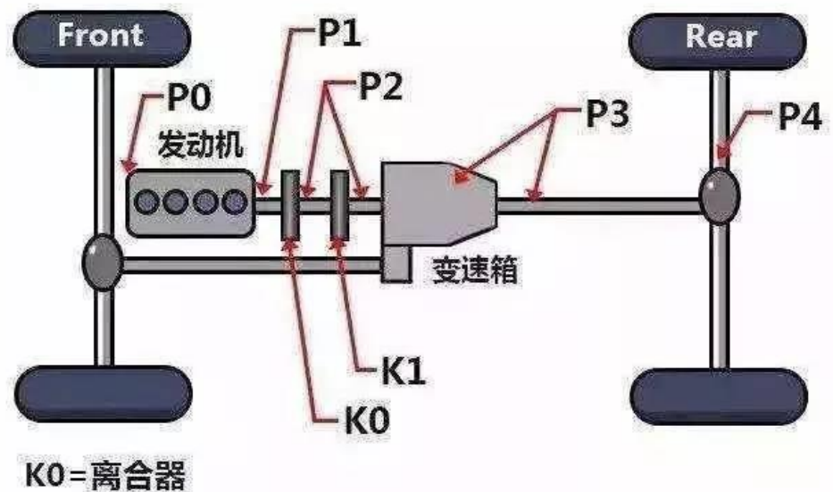
图表 11：混动电机位置示意图
