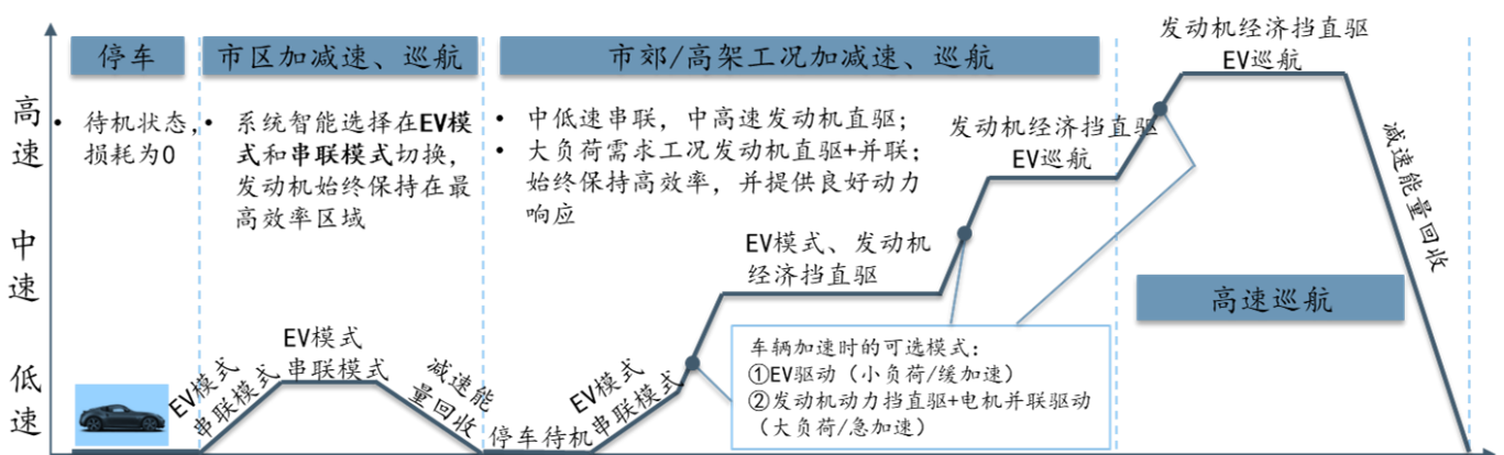
图表 20：柠檬 DHT 工作模式
