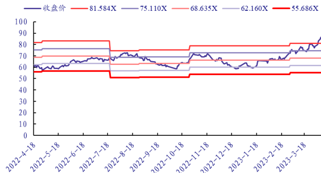
图 5: PE-Bands
