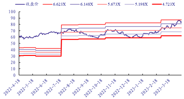
图 6: PB-Bands
