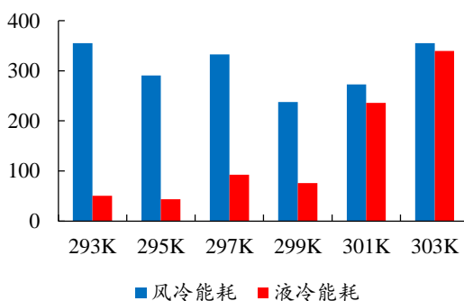
图33：液冷能耗相比风冷能耗更低
