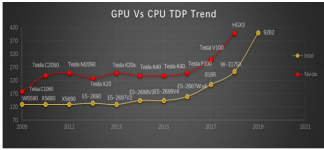
图13: GPU与CPU的热设计功耗均呈现上升趋势
