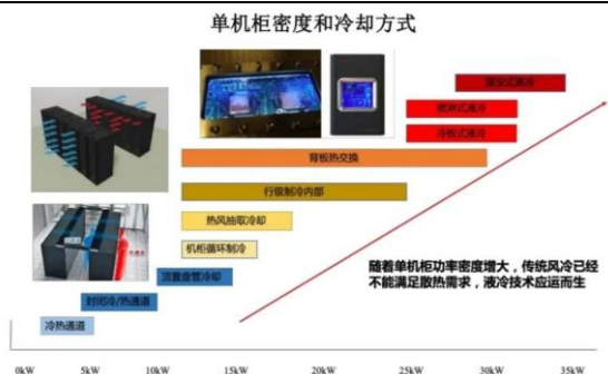
图16: 更高单机柜功率密度催化更优温控解决方案
