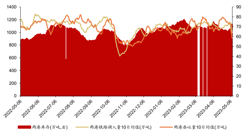
图3: 秦皇岛港及曹妃甸港煤炭库存及吞吐情况
