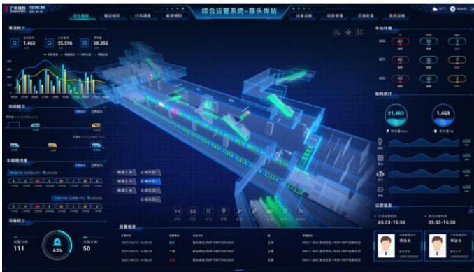
图23: 以华佳 Mos 为底座的新一代综合监控系统（应用于广州地铁 18 号线）
