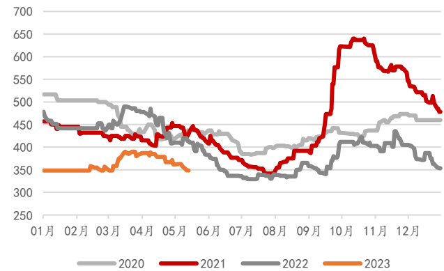
图表13：华中水泥(P.O42.5散装)价格(元/吨)分年度
