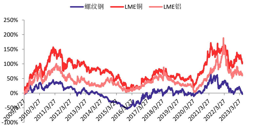
图 4: 原材料价格变动率
