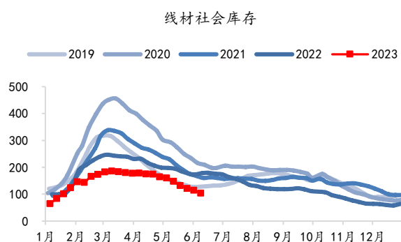
图表 76 线材社会库存 (万吨)
