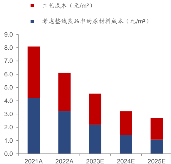
图表：PET铜箔成本拆分
