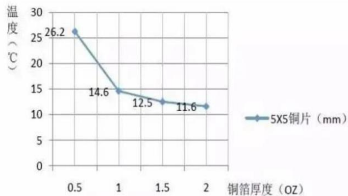
图表: 传统铜箔与复合铜箔安全性对比
