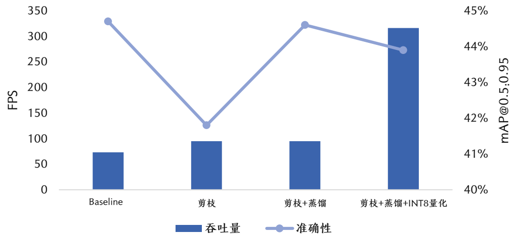
图 4: 目标检测 YOLOv5m 模型优化测试结果
